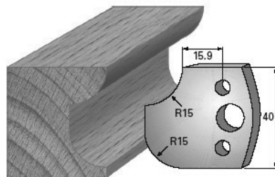
SP-Messer/Blade = Art.-Nr./Item no. 36177 HS-Messer/Blade = Art.-Nr./Item no. 36477 Abweiser/Deflector = Art.-Nr./Item no. 37177
