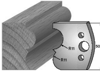
SP-Messer/Blade = Art.-Nr./Item no. 38572 HS-Messer/Blade = Art.-Nr./Item no. 36572 Abweiser/Deflector = Art.-Nr./Item no. 39572
