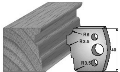
SP-Messer/Blade = Art.-Nr./Item no. 3639 HS-Messer/Blade = Art.-Nr./Item no. 36339 Abweiser/Deflector = Art.-Nr./Item no. 3739
