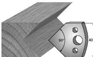
SP-Messer/Blade = Art.-Nr./Item no. 36127 HS-Messer/Blade = Art.-Nr./Item no. 36427 Abweiser/Deflector = Art.-Nr./Item no. 37127
