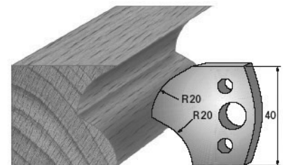
SP-Messer/Blade = Art.-Nr./Item no. 36120 HS-Messer/Blade = Art.-Nr./Item no. 36420 Abweiser/Deflector = Art.-Nr./Item no. 37120
