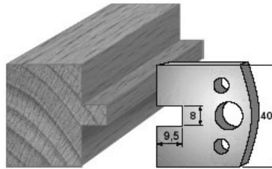
SP-Messer/Blade = Art.-Nr./Item no. 3695 HS-Messer/Blade = Art.-Nr./Item no. 36395 Abweiser/Deflector = Art.-Nr./Item no. 3795
