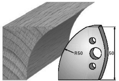
SP-Messer/Blade = Art.-Nr./Item no. 38567 HS-Messer/Blade = Art.-Nr./Item no. 36567 Abweiser/Deflector = Art.-Nr./Item no. 39567
