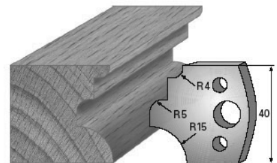
SP-Messer/Blade = Art.-Nr./Item no. 36129 HS-Messer/Blade = Art.-Nr./Item no. 36429 Abweiser/Deflector = Art.-Nr./Item no. 37129
