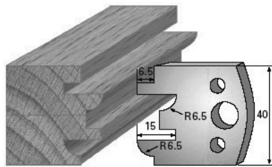
SP-Messer/Blade = Art.-Nr./Item no. 3696 - Konter 1 HS-Messer/Blade = Art.-Nr./Item no. 36396 Abweiser/Deflector = Art.-Nr./Item no. 3796
