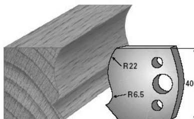
SP-Messer/Blade = Art.-Nr./Item no. 36128 HS-Messer/Blade = Art.-Nr./Item no. 36428 Abweiser/Deflector = Art.-Nr./Item no. 37128
