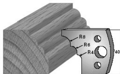
SP-Messer/Blade = Art.-Nr./Item no. 36133 HS-Messer/Blade = Art.-Nr./Item no. 36433 Abweiser/Deflector = Art.-Nr./Item no. 37133
