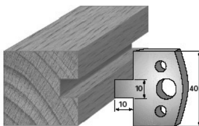
SP-Messer/Blade = Art.-Nr./Item no. 3691 HS-Messer/Blade = Art.-Nr./Item no. 36391 Abweiser/Deflector = Art.-Nr./Item no. 3791
