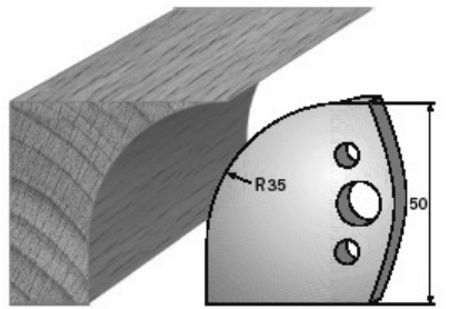
SP-Messer/Blade = Art.-Nr./Item no. 38564 HS-Messer/Blade = Art.-Nr./Item no. 36564 Abweiser/Deflector = Art.-Nr./Item no. 39564
