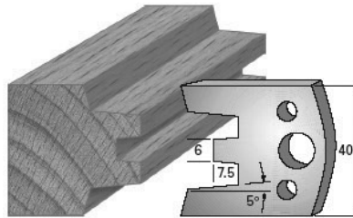
SP-Messer/Blade = Art.-Nr./Item no. 36113 HS-Messer/Blade = Art.-Nr./Item no. 36413 Abweiser/Deflector = Art.-Nr./Item no. 37113
