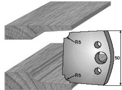
SP-Messer/Blade = Art.-Nr./Item no. 38579 HS-Messer/Blade = Art.-Nr./Item no. 36579 Abweiser/Deflector = Art.-Nr./Item no. 39579
