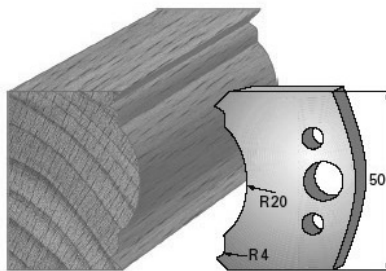
SP-Messer/Blade = Art.-Nr./Item no. 38507 HS-Messer/Blade = Art.-Nr./Item no. 36507 Abweiser/Deflector = Art.-Nr./Item no. 39507
