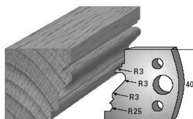
SP-Messer/Blade = Art.-Nr./Item no. 36122 HS-Messer/Blade = Art.-Nr./Item no. 36422 Abweiser/Deflector = Art.-Nr./Item no. 37122
