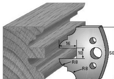
SP-Messer/Blade = Art.-Nr./Item no. 38523 HS-Messer/Blade = Art.-Nr./Item no. 36523 Abweiser/Deflector = Art.-Nr./Item no. 39523
