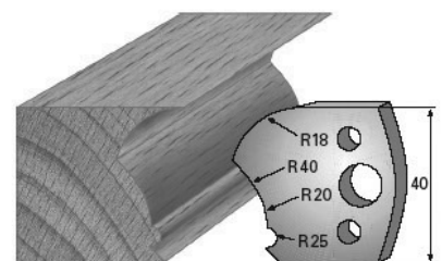
SP-Messer/Blade = Art.-Nr./Item no. 36123 HS-Messer/Blade = Art.-Nr./Item no. 36423 Abweiser/Deflector = Art.-Nr./Item no. 37123
