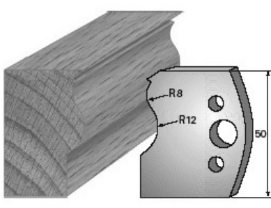
SP-Messer/Blade = Art.-Nr./Item no. 38578 HS-Messer/Blade = Art.-Nr./Item no. 36578 Abweiser/Deflector = Art.-Nr./Item no. 39578
