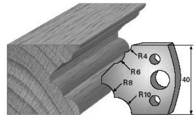
SP-Messer/Blade = Art.-Nr./Item no. 36126 HS-Messer/Blade = Art.-Nr./Item no. 36426 Abweiser/Deflector = Art.-Nr./Item no. 37126
