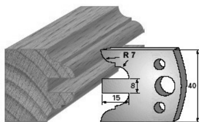
SP-Messer/Blade = Art.-Nr./Item no. 3698 - Konter 3 HS-Messer/Blade = Art.-Nr./Item no. 36398 Abweiser/Deflector = Art.-Nr./Item no. 3798
