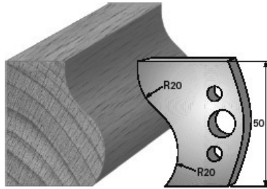
SP-Messer/Blade = Art.-Nr./Item no. 38571 HS-Messer/Blade = Art.-Nr./Item no. 36571 Abweiser/Deflector = Art.-Nr./Item no. 39571
