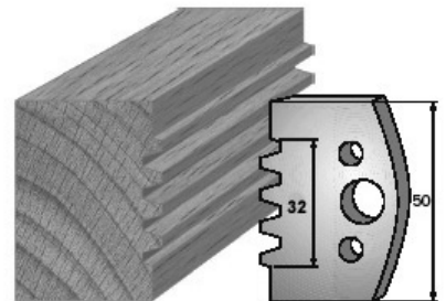
SP-Messer/Blade = Art.-Nr./Item no. 38576 HS-Messer/Blade = Art.-Nr./Item no. 36576 Abweiser/Deflector = Art.-Nr./Item no. 39576
