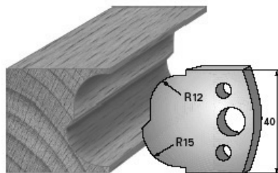
SP-Messer/Blade = Art.-Nr./Item no. 36115 HS-Messer/Blade = Art.-Nr./Item no. 36415 Abweiser/Deflector = Art.-Nr./Item no. 37115
