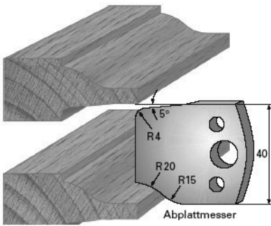
Abplattmesser
