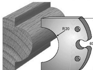
SP-Messer/Blade = Art.-Nr./Item no. 60016 HS-Messer/Blade = Art.-Nr./Item no. 62016 Abweiser/Deflector = Art.-Nr./Item no. 61016
